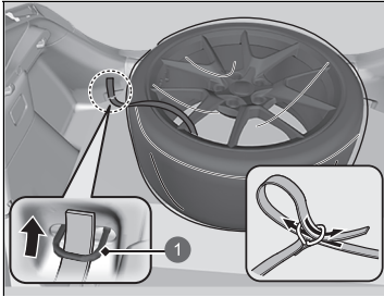
1 Ancoraggio posteriore
