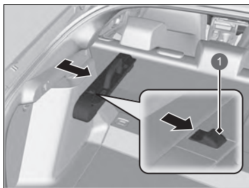
1 Leva
